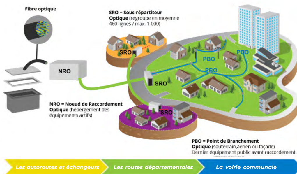
SCHÉMA DU RÉSEAU FIBRE OPTIQUE ROSACE
